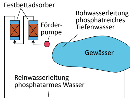
Phosphatentfernung mit einem FerroSorp® GW - Festbettadsorber
